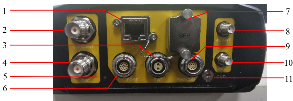
图 2-3 后面板
